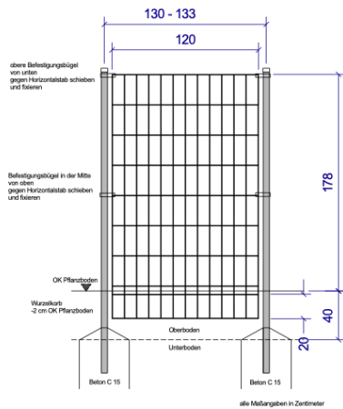
Abbildung 4 Systemskizze für den Einbau und Unterkonstruktion der laufenden Hecke, individuelle Halterungen bei der Schatteninsel
